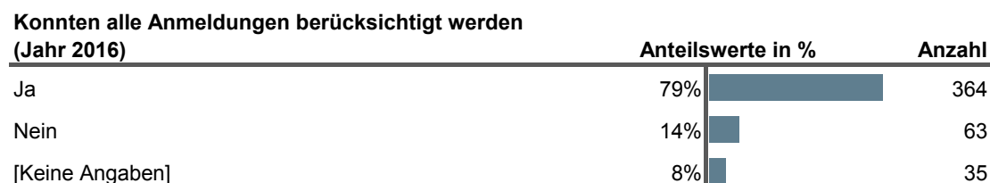
Abbildung 3-8: SEB: Nachfrageüberschuss
